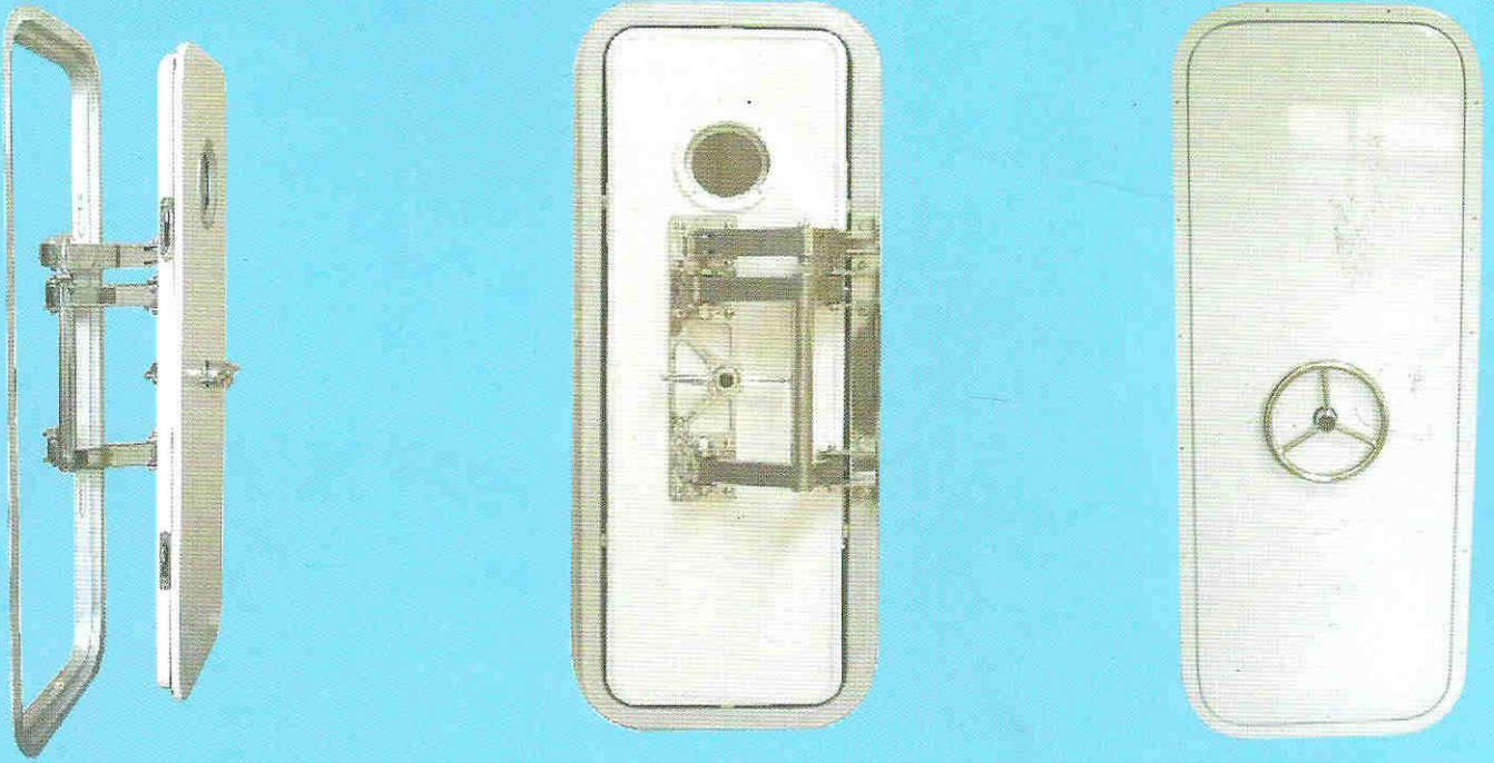
Watertight Pantograf 4 - 6 Mekanizmalı Uzaktan Kumandalı Kilitleme Sistem
